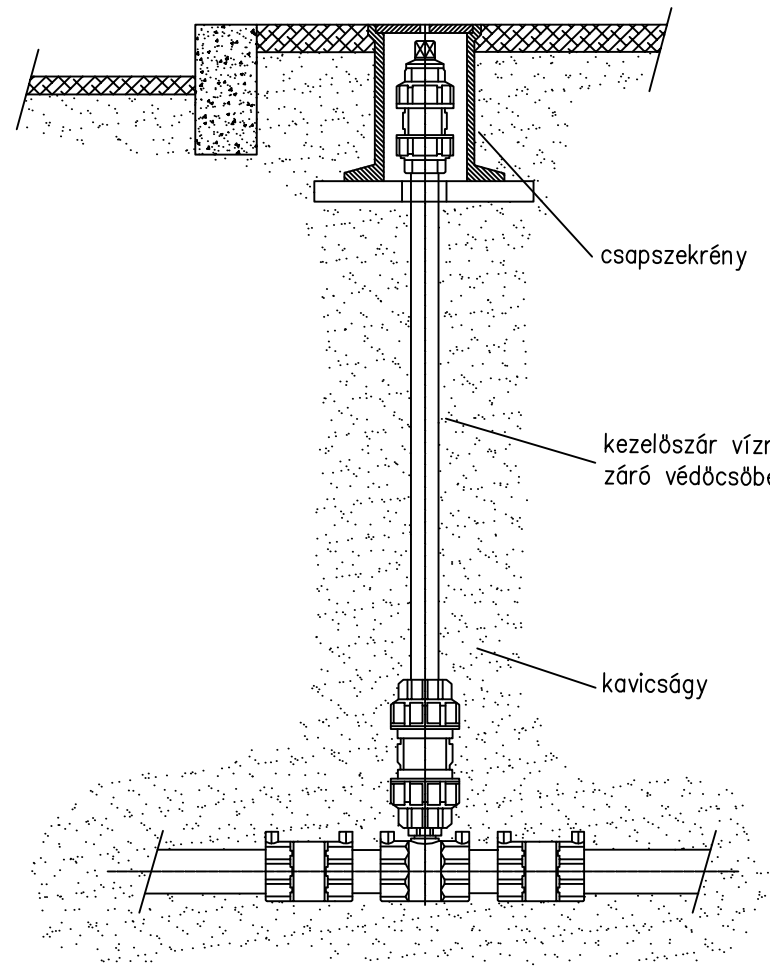
Műanyag gömbcsap beépítése M1:15
